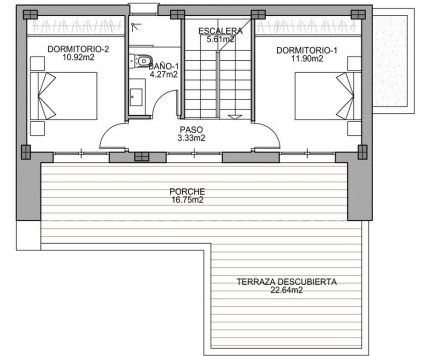
PLANTA PRIMERA
